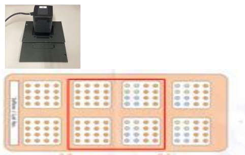
ELISA 法にてサイトカインを検出するチップ（下）と検出カメラ（上）
